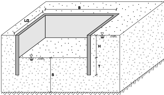
Abbildung 2. Systemskizze einer Baugrube mit den zugehörigen geometrischen Abmessungen.
