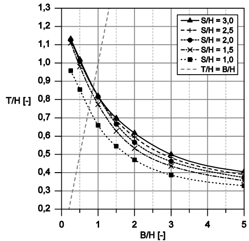
Abbildung 4. Bemessungsdiagramm für die Stirnseite in homogenem, isotropem Baugrund.
