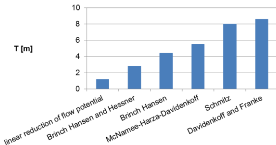
Abbildung 1. Erforderliche Einbindetiefe T auf Grundlage verschiedener Näherungslösungen für eine Baugrube der Breite B = 10 m mit einer Wasserspiegeldifferenz von H = 10 m.
