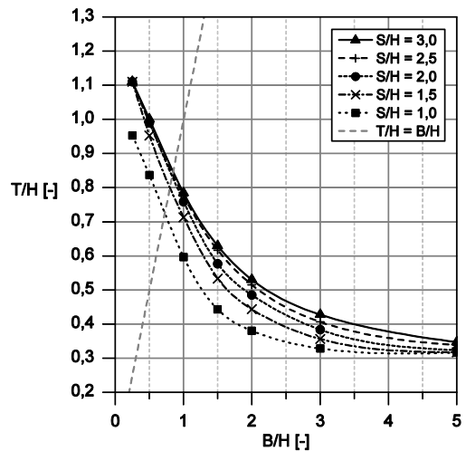
Abbildung 5. Bemessungsdiagramm für die Längsseite in homogenem, isotropem Baugrund.
