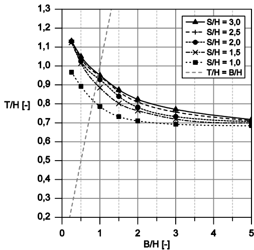
Abbildung 3. Bemessungsdiagramm für den Eckbereich in homogenem, isotropem Baugrund.
