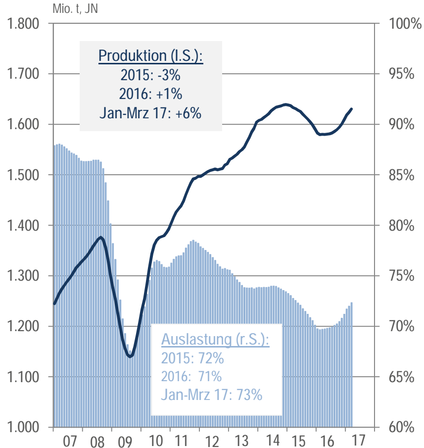
Welt-Rohstahlproduktion und Auslastung (12-Monatsdurchschnitte)
