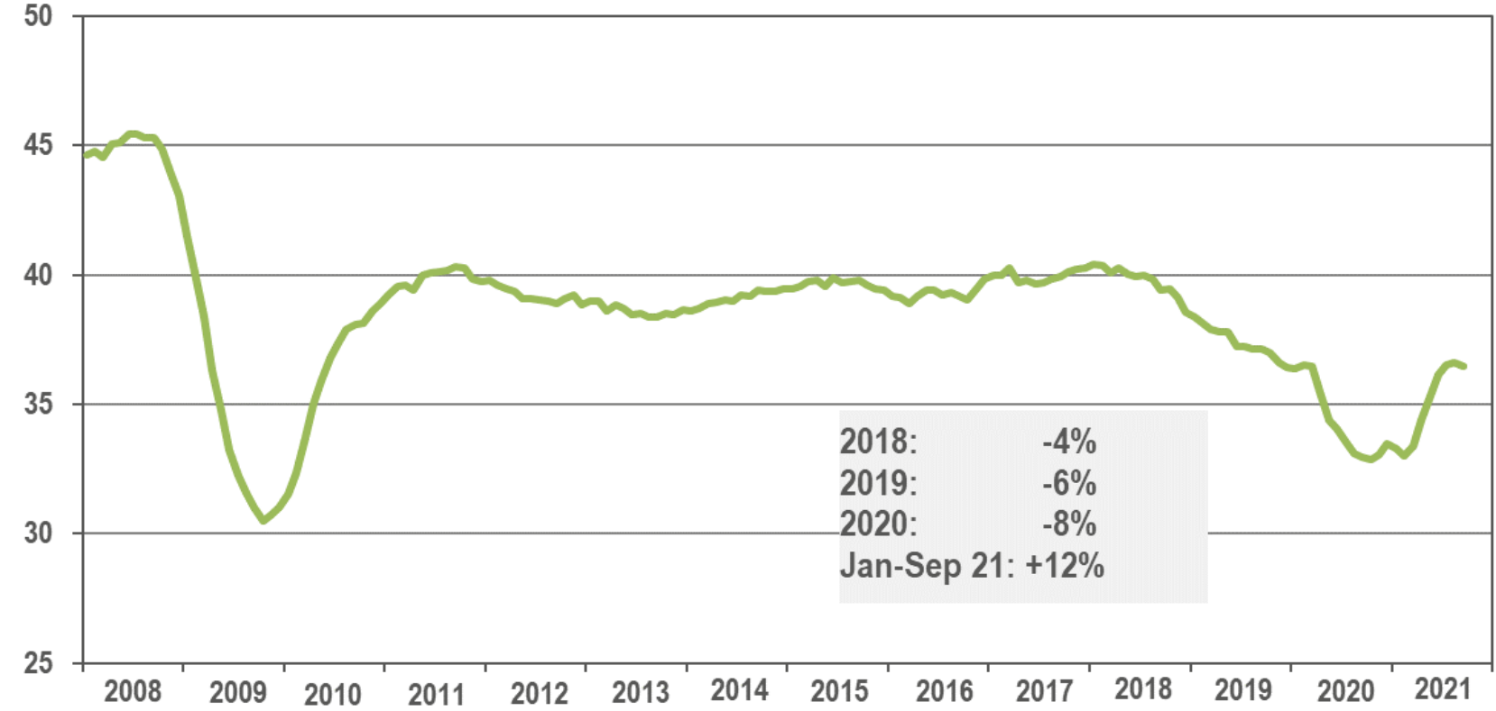
Lieferungen Walzstahl (Millionen Tonnen, 12MD, annualisiert)
